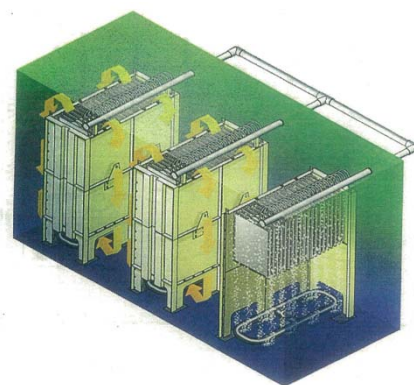
膜ユニット設置例
